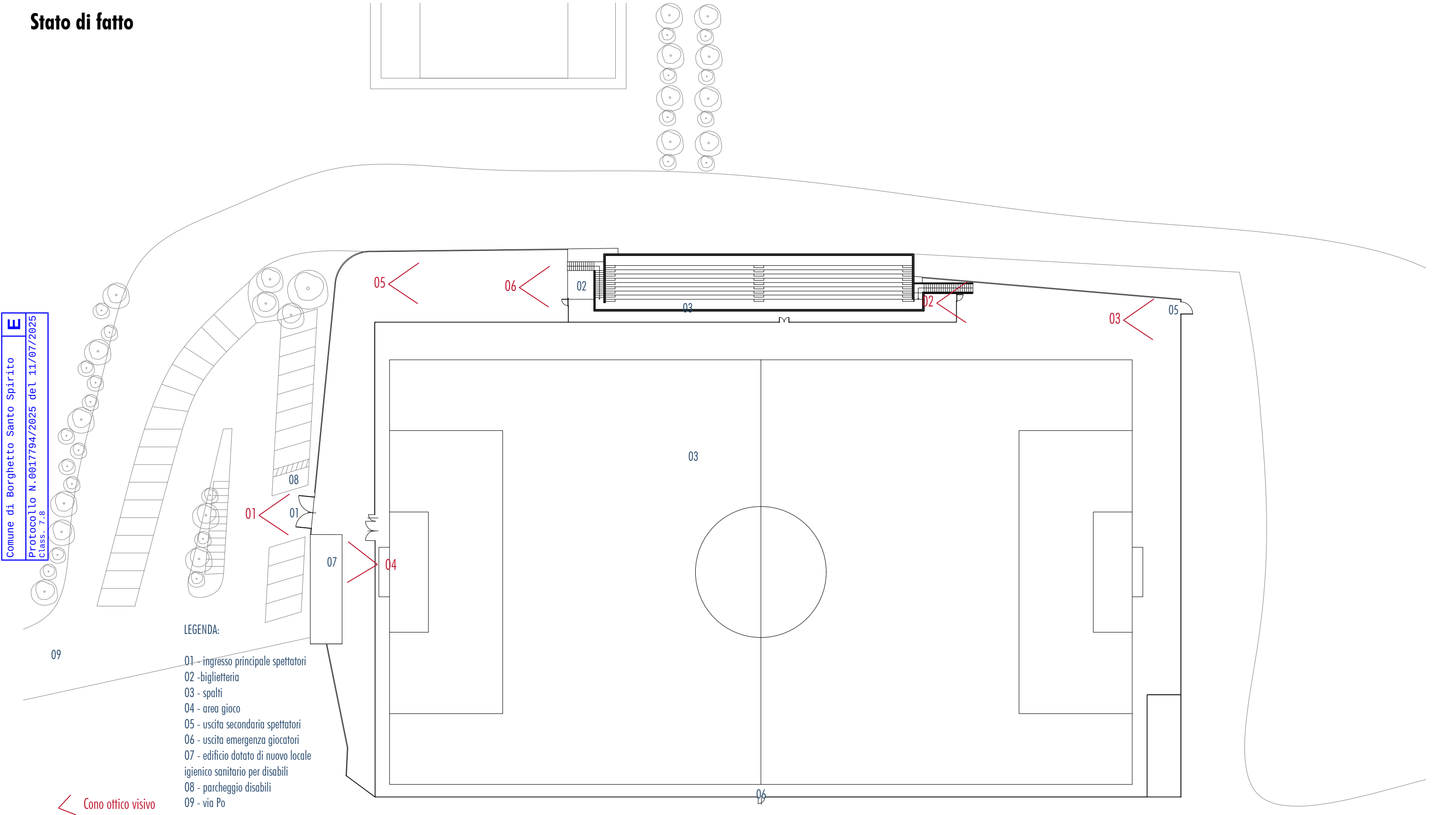
Campo sportivo Oliva - Pianta livello 0 - scala 1: 500
