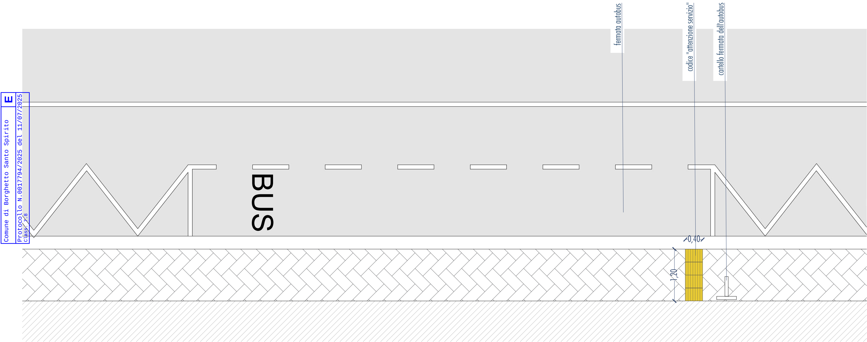
Soluzione progettuale tipo con segnaletica per ipovedenti per fermata autobus
