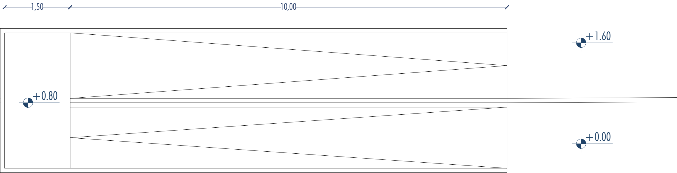
Soluzione progettuale tipo per persone con mobilità ridotta, esempio rampa doppia con pendenza pari a 8%
