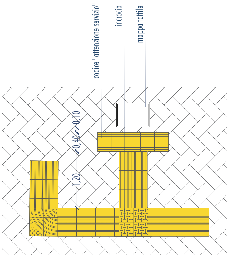
Soluzione progettuale tipo con segnaletica per ipovedenti per accedere al pannello informativo
