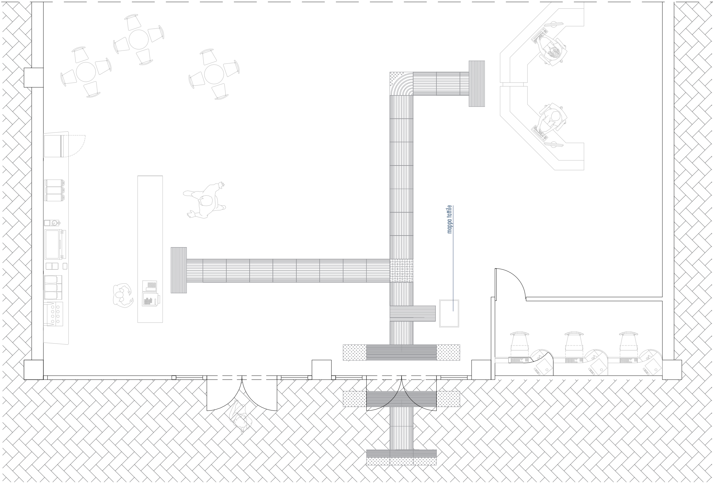
Soluzione progettuale tipo per ingresso ad edificio aperto al pubblico con segnaletica per ipovedenti
