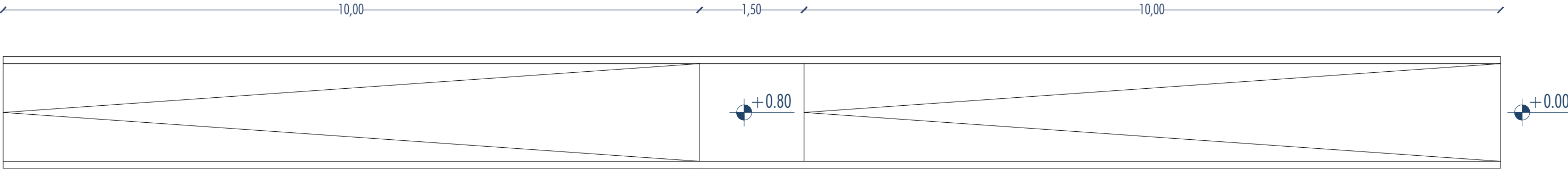
Soluzione progettuale tipo per persone con mobilità ridotta, esempio rampa lineare con pendenza pari a 8%
