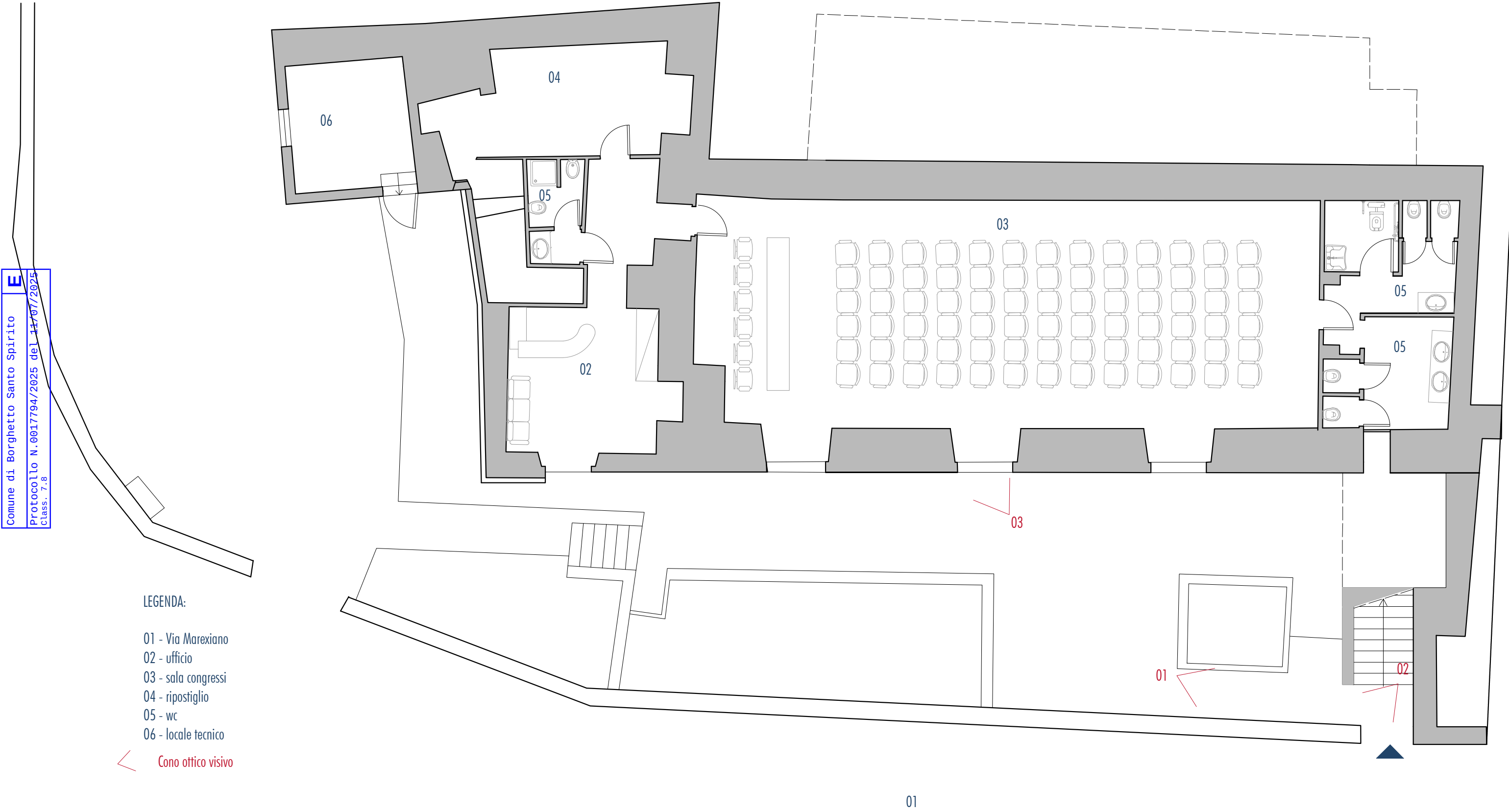
Palazzo Marexiano - Pianta livello 0 - scala 1:100
