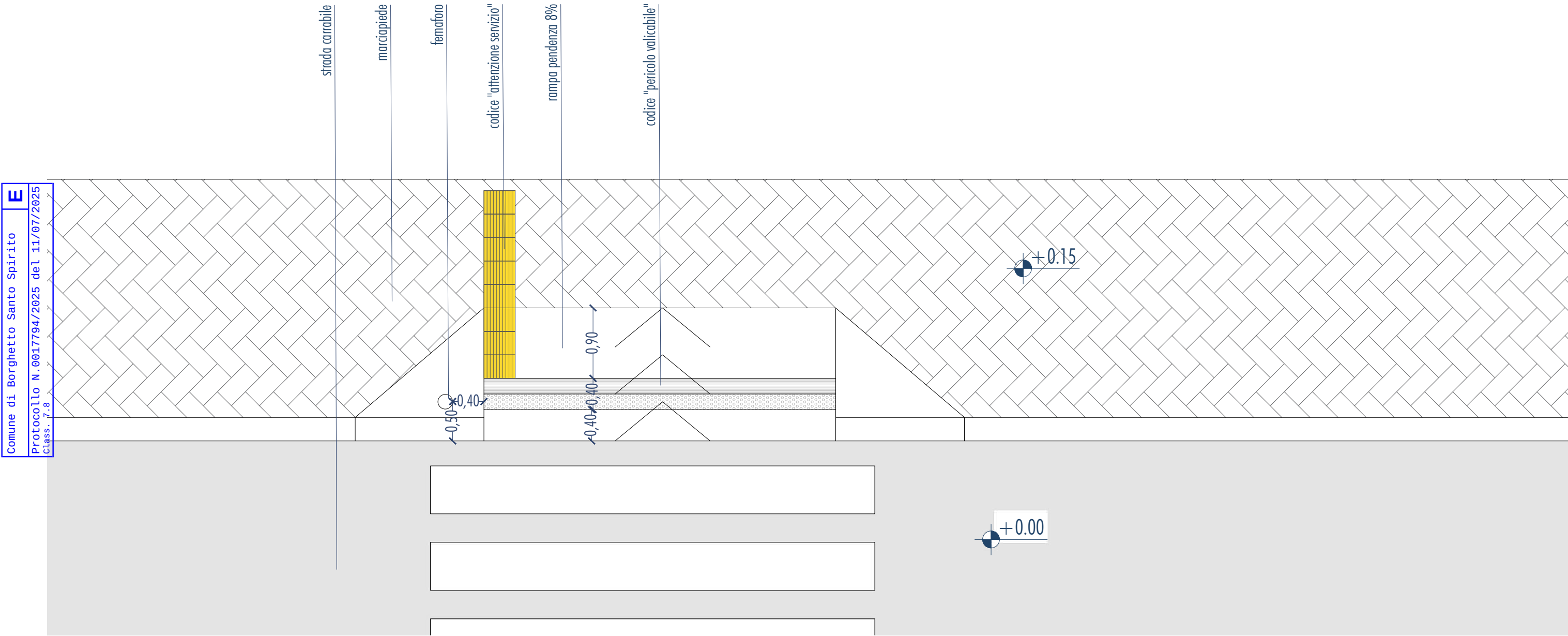
Soluzione progettuale tipo con segnaletica per ipovedenti e per persone con mobilità ridotta per attraversamento pedonale
