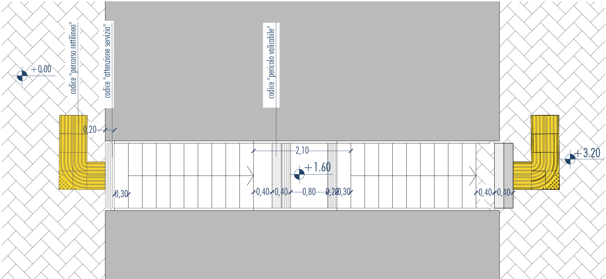
Soluzione progettuale tipo con segnaletica per ipovedenti per scala
