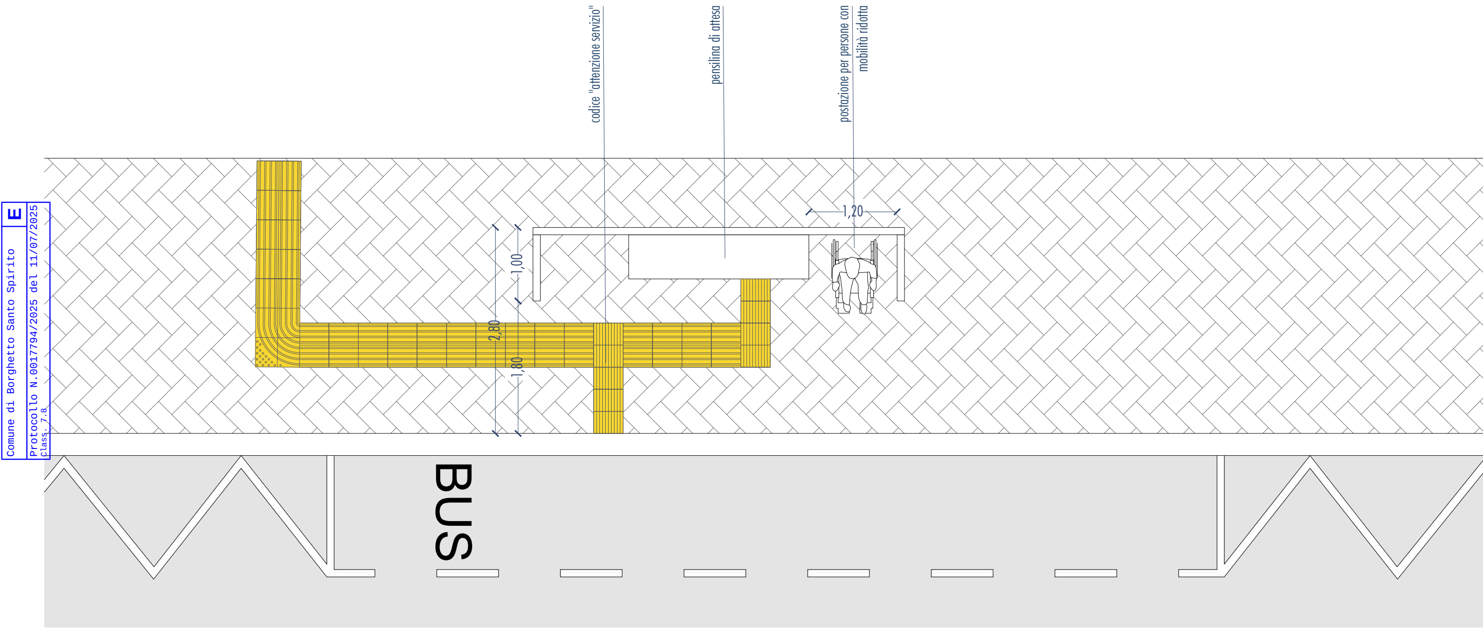
Soluzione progettuale tipo con segnaletica per ipovedenti e per persone con mobilità ridotta per fermata autobus
